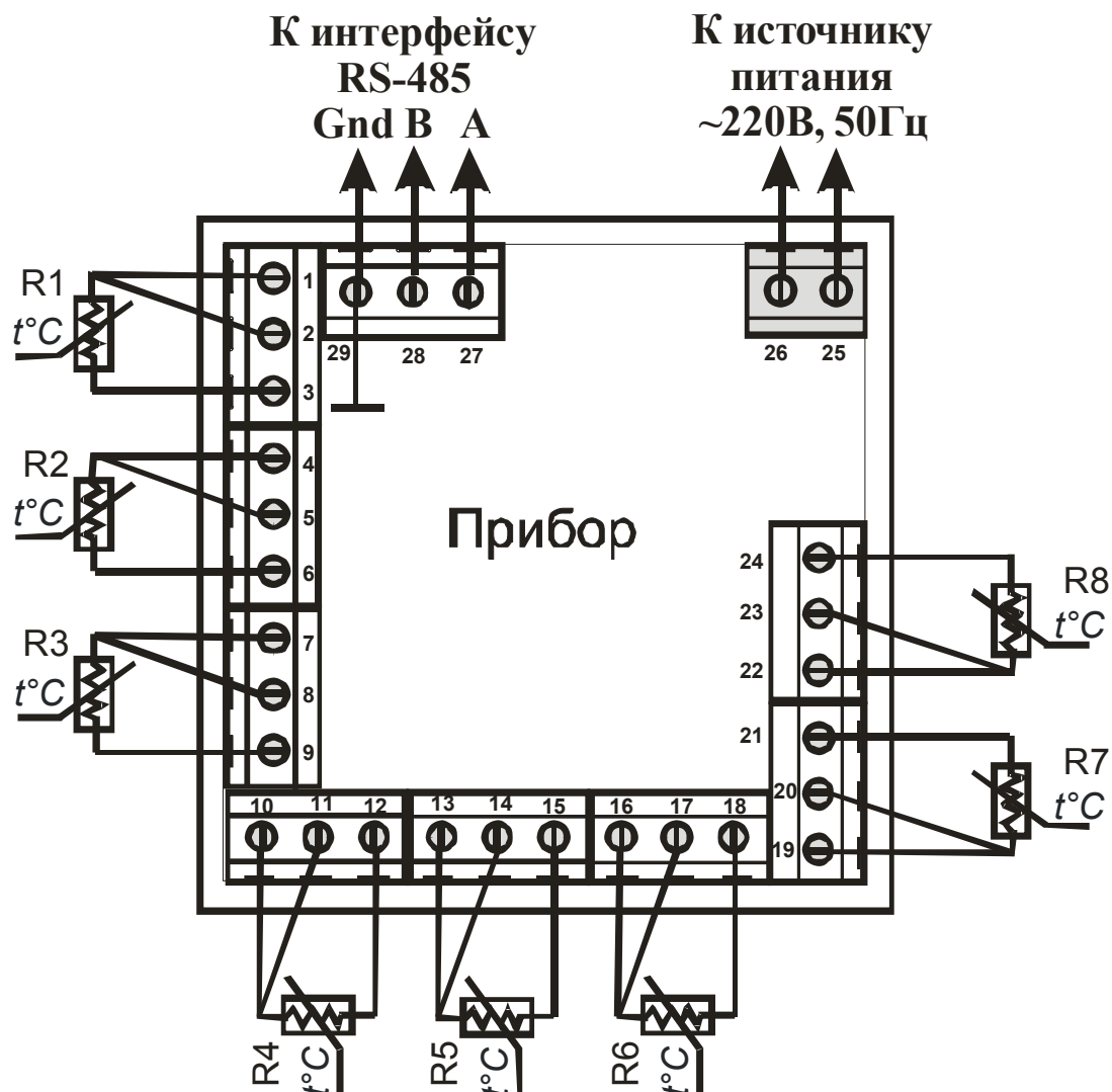
Рисунок 8.1 – Схема подключения ТС, интерфейса связи и источника питания
