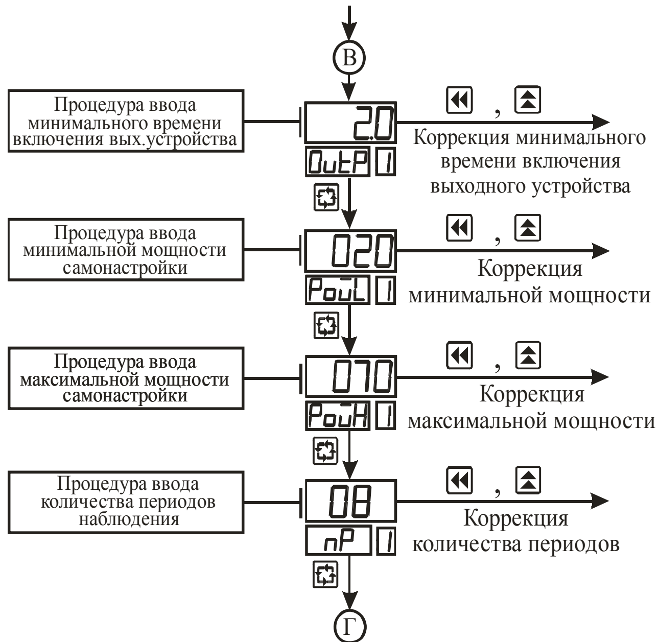
Рисунок 3.12 – Схема алгоритма работы в режиме “Константы ПИД” (продолжение)
